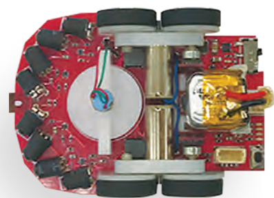
<原寸> 2018年マイクロマウス競技優勝機 「Fantom2nd(松井 祐樹氏)」 長さ52mm x 幅38mm x 高さ20mm 重量11.8g
